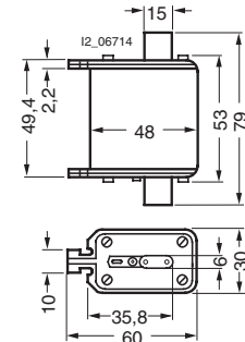
3NE1 02...-0, 3NE1 02...-2, 3NE8 0...-1
