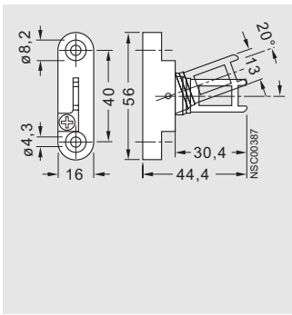
3SX3 254 radius actuator
