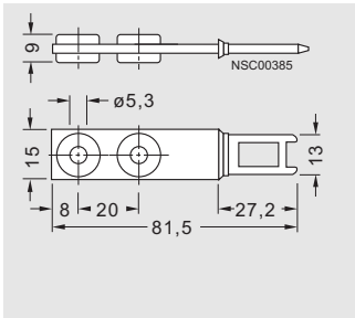
3SX3 254 radius actuator
